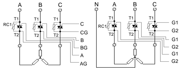
图 7: C3、K6 型应用 三相三线制移相触发
