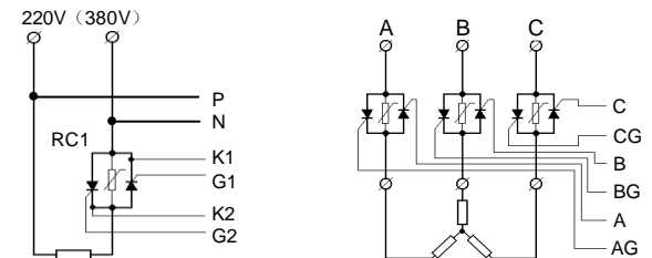
图 11: C2 型应用二 传统触发型单路移相触发
