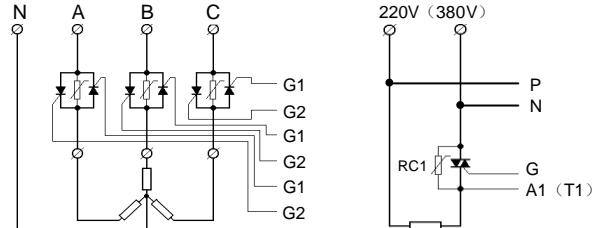
图 10: C2 型应用一 传统触发型单路移相触发
