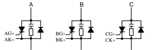
图 13: C6 半控型应用。单硅二极管反并联，Y/Δ形接法。自动适应相序。 如果采用单硅和二极管反并联，则不接图中三个辅助组件
