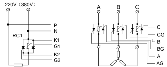
图 11: C2 型应用二 传统触发型单相移相触发
