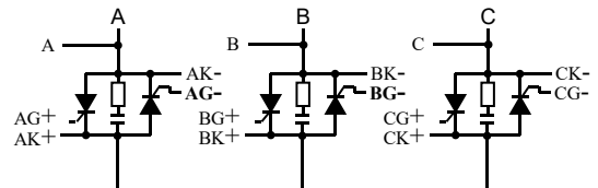
图 14: C7 型应用。单硅反并联, Y/Δ 接法。自动适应相序。如果采用单硅和二极管反并联, 则不按图中三个辅助组件
