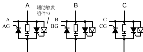
图 14: C7 型应用。单硅反并联, Y/Δ 接法。自动适应相序。如果采用单硅和二极管反并联, 则不按图中三个辅助组件
